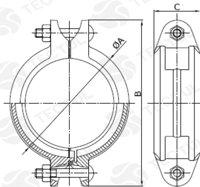
* Vista de sección transversal de tipo informativa. No representa versión específica en la Unión.
