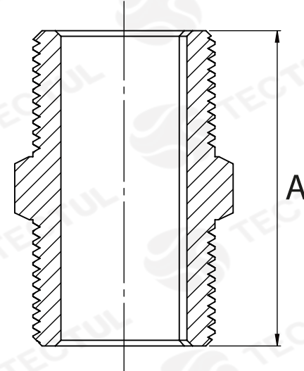
* Vista de sección transversal de tipo informativa. No representa versión específica del accesorio.
