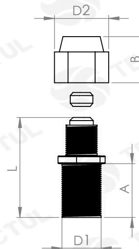
* Vista de sección transversal de tipo informativa. No representa versión específica del accesorio.
