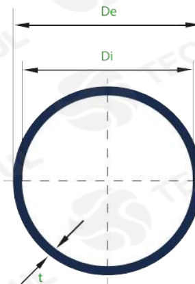
Class RDE 11 / PN10 / Serie 5
